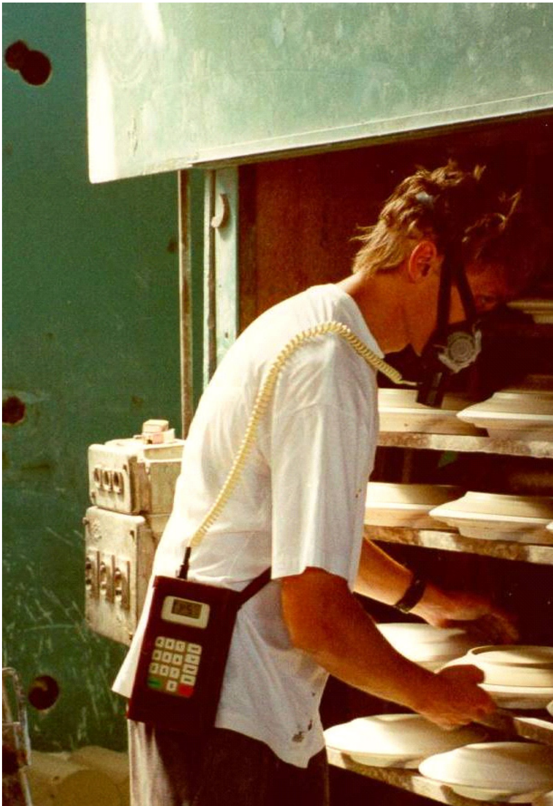
Fot. 1. Pomiar wydatku energetycznego na stanowisku pracy miernikiem MWE
