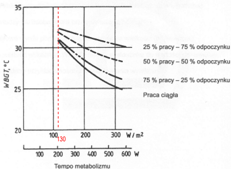
Rys. 1. Krzywe wartości dopuszczalnych wskaźnika WBGT
